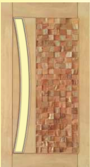
PORTA AMÉRICA PARA VIDRO EM ARCO CÓDIGO 2898 - 2,10m x 0,72m CÓDIGO 2899 - 2,10m x 0,82m CÓDIGO 2900 - 2,10m x 0,92m CÓDIGO 2901 - 2,10m x 1,02m CÓDIGO 2902 - 2,10m x 1,12m CÓDIGO 2903 - 2,10m x 1,22m
