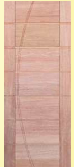
PORTA PIVOTANTE BBB-R FRISO EM ARCO CÓDIGO 2021 - 2,10m x 0,62m CÓDIGO 2022 - 2,10m x 0,72m CÓDIGO 2023 - 2,10m x 0,82m CÓDIGO 2024 - 2,10m x 0,92m CÓDIGO 2025 - 2,10m x 1,02m CÓDIGO 2026 - 2,10m x 1,12m CÓDIGO 2027 - 2,10m x 1,22m
