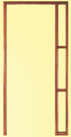
BATENTE SACI P/V RETO CÓDIGO 6028 - 0,82m x 1,04m CÓDIGO 6029 - 0,92m x 1,14m
