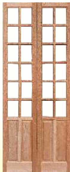
PORTA CAMARÃO 2 ALMOF. 12 VIDROS CÓDIGO 3064 - 2,10m x 0,62m CÓDIGO 3065 - 2,10m x 0,72m CÓDIGO 3066 - 2,10m x 0,82m CÓDIGO 3067 - 2,10m x 0,92m
